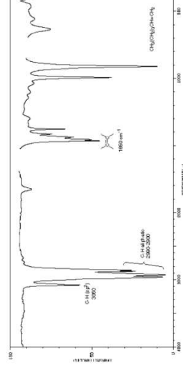
Hexene
