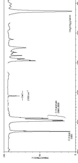
Hexyne
