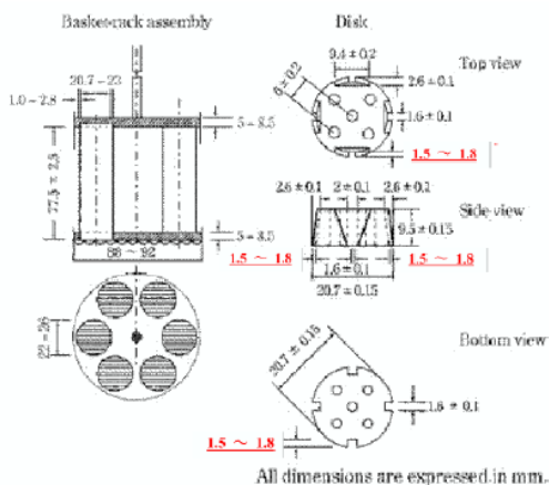
Fig. 6.09-1 Disintegration apparatus
