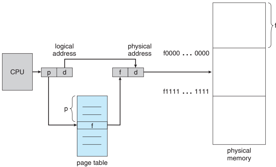
Figure 7.7 Paging hardware.
