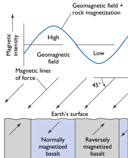
(d) MAGNETIC ANOMALIES
