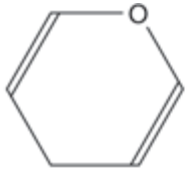
Pyran
